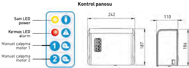
Kontrol panosu
