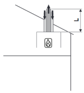
C33 Uygulama Örneği
