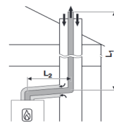
C93 Uygulama Örneği
